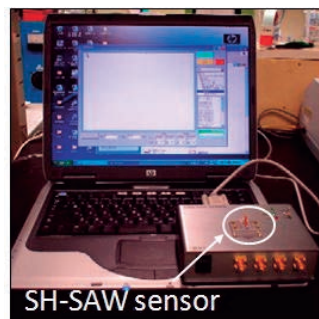
図5 開発した小型液体計測装置。
