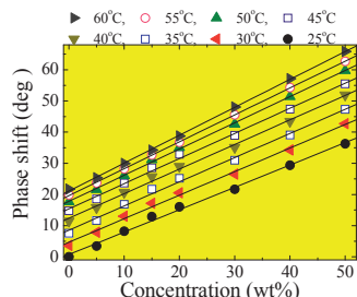
図3 温度を変化させたメタノール水溶液測定。
