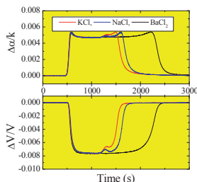
図4 液体自動計測装置を用いた電界質水溶液評価。過渡応答よりイオン判別が可能。
